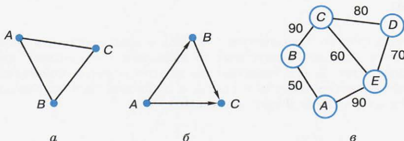
Рис. 1.6. Графы
