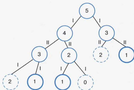
Рис. 1.11. Дерево игры
