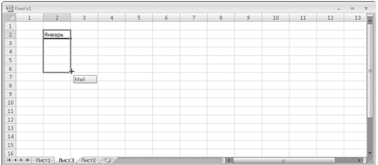
Рис. 2.2. Процесс автозаполнения
