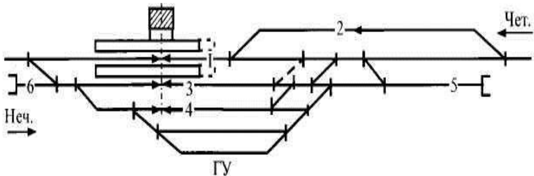
Рис. 3.5. Схема промежуточной станции на однопутной линии с полу-продольным расположением путей
