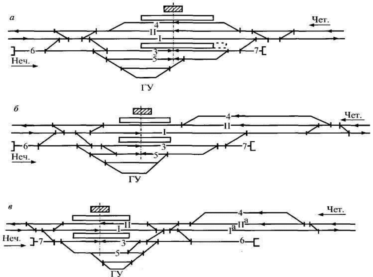
Рис. 3.7. Схемы промежуточных станций на двухпутной линии с расположением путей: a — поперечным; b — полупродольным; в — продольным
