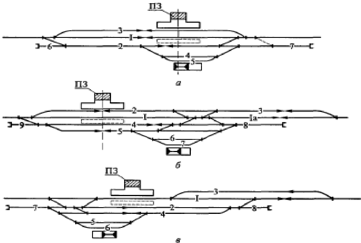
Рис. 26. Принципиальные схемы промежуточных станций однопутных линий с поперечным (а), продольным (б) и полупродольным (в) расположением приемоотправочных путей:
